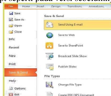
Gambar 3. Meyimpan Data
